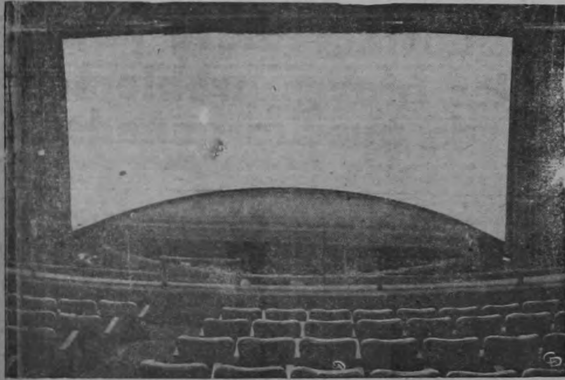
Esta pantalla de Cinerama, instalada en un Teatro de Broadway en Nueva York, tiene tres secciones principales. Consiste de más de 1.000 tiras de cinta plástica, dispuestas en forma similar a las hojas de una persiana tipo veneciano.
